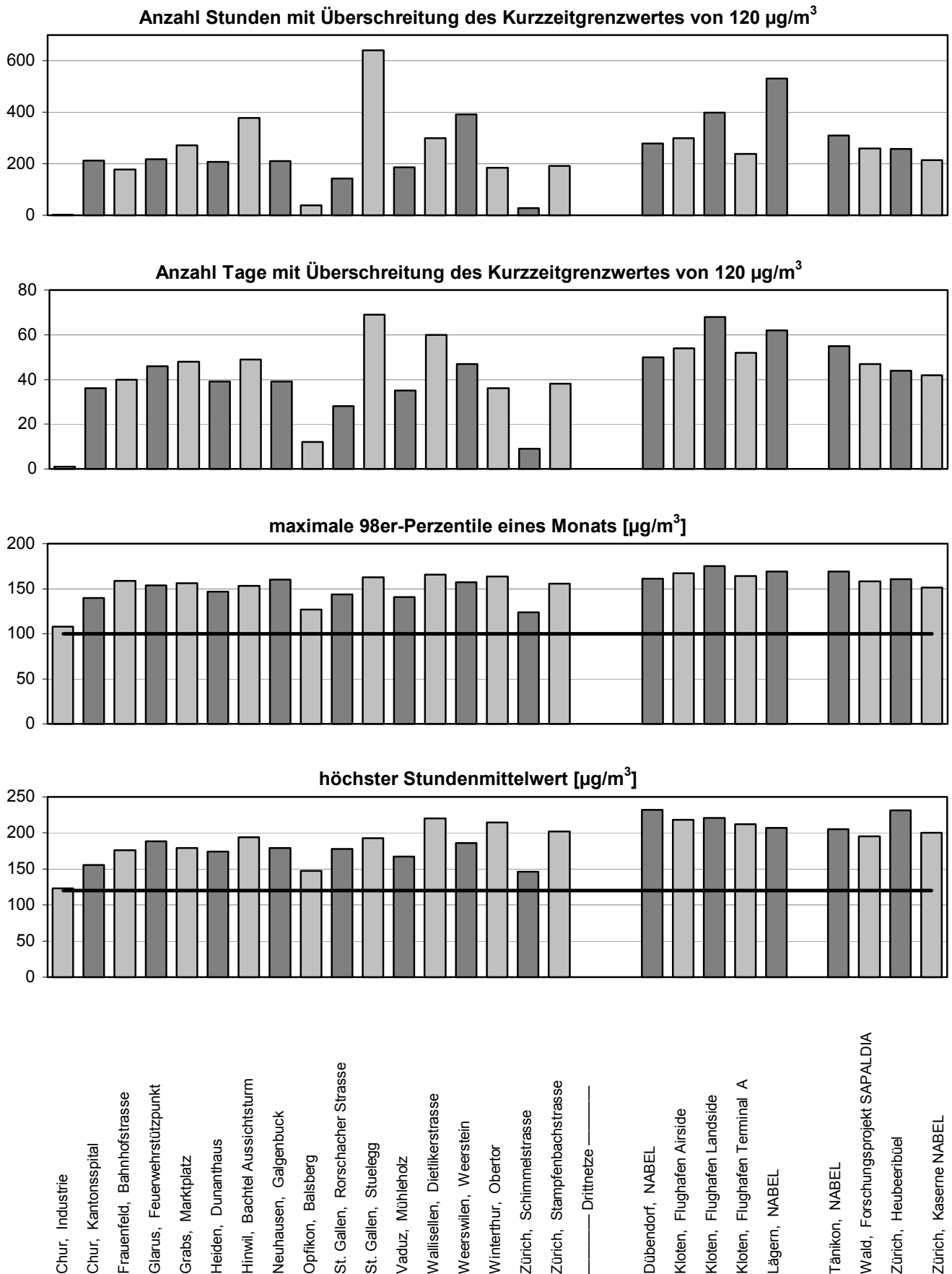
Abb. 8: Kennwerte der Ozon-Belastung 2002 an den automatischen Messstationen im OSTLUFT-Gebiet ( ——— Grenzwerte)
