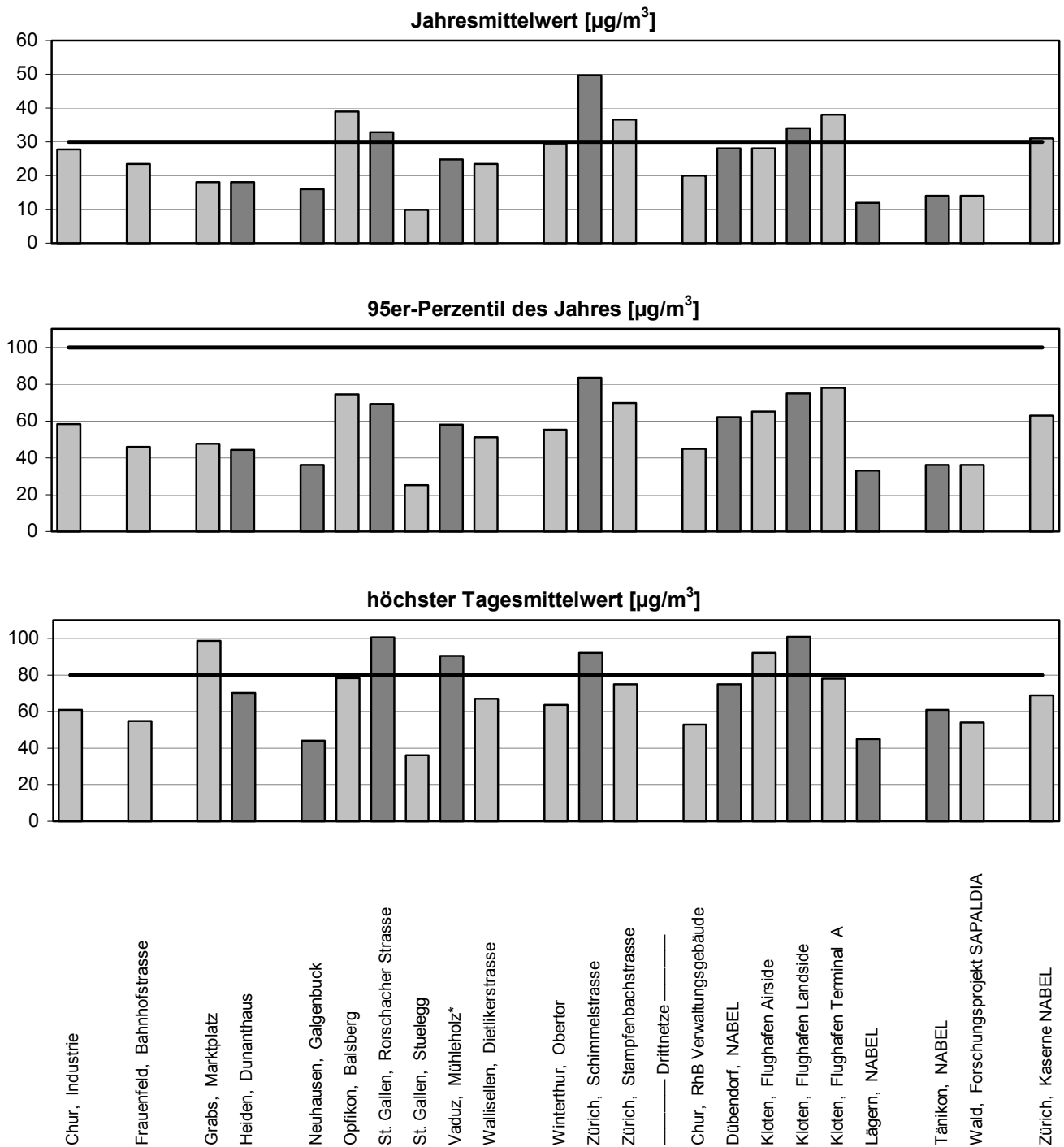
Abb. 7: Kennwerte der NO 2 -Belastung 2002 an den automatischen Messstationen im OSTLUFT-Gebiet ( ——— Grenzwerte)
